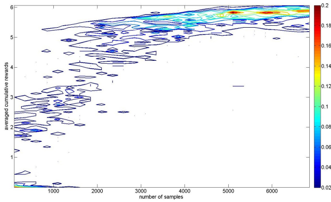
Fig. 8. Wet-chicken.
